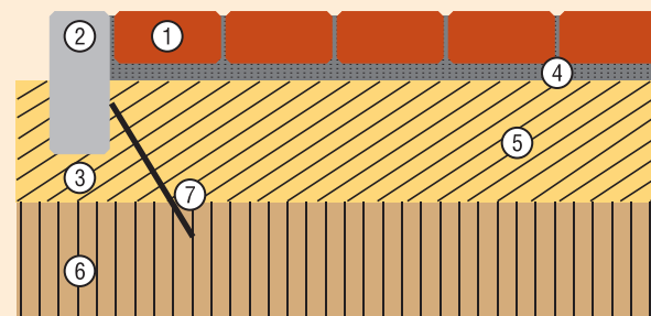
Рисунок №3. Водоотвод из монтажного слоя.
